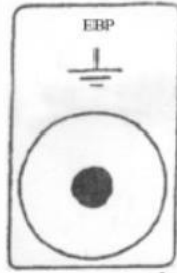
图2 接地连接点符号式样
